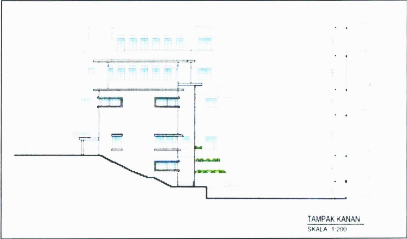
Gambar 20. Tampak Kanan Villa Isola Sumber: Dwiwandana (2023)
